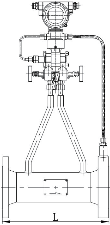
图 7 法兰钻孔角接取压式 (KF)
