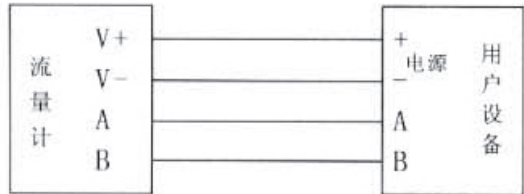
图 11 RS485 通讯
