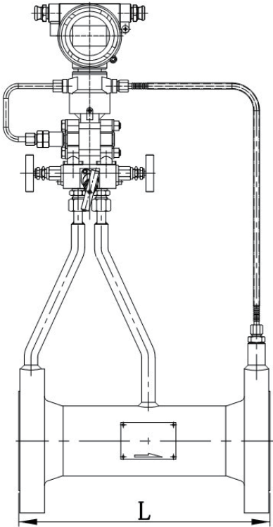
图 6 孔板取压环整体角接取压式 (KH)
