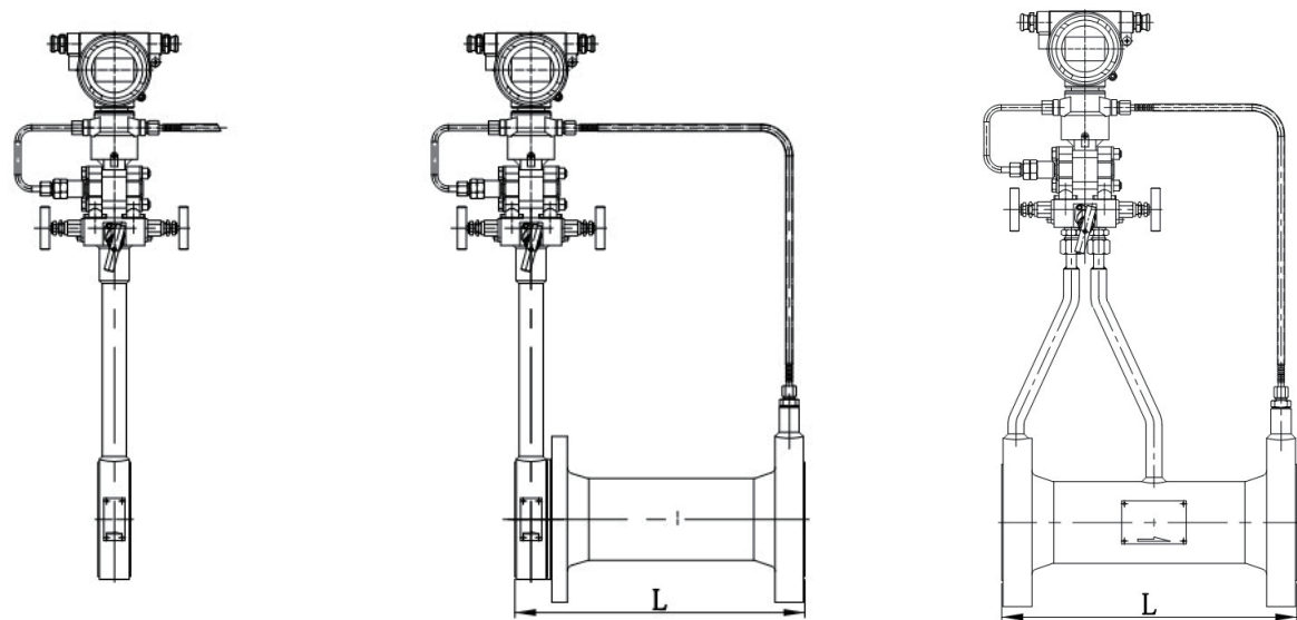
图 3 TDF-II-K 型一体化标准孔板 图 4 TDF-II-W 型一体化文丘里 图 5 TDF-II-X 型一体化楔形孔板
