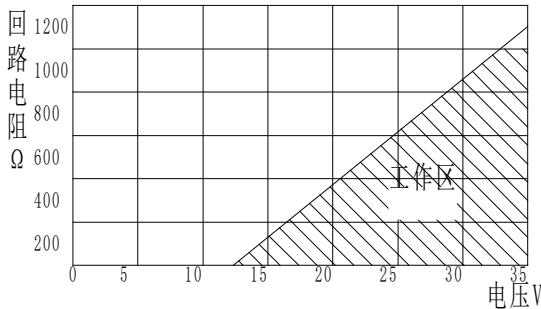
图 9 电路电压与回路电阻关系图
