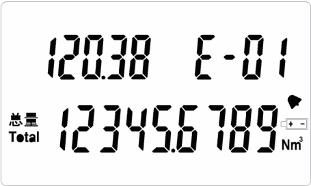
图 18 报警屏
