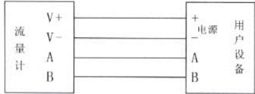
图 12 HART 通讯
