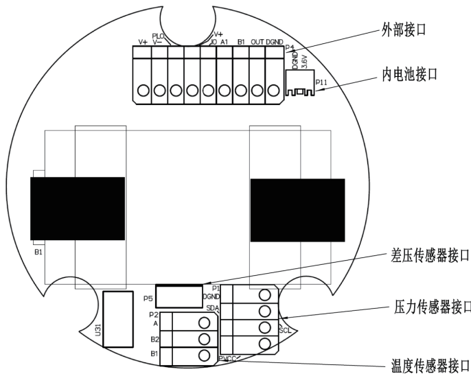
图 13 内部接线图
